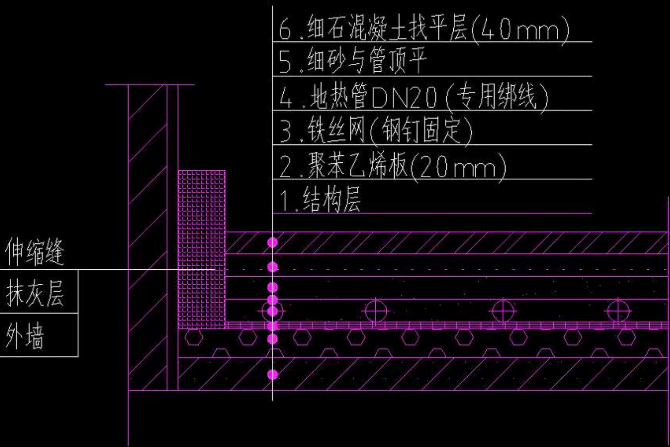
标准层辐射供暖地板的构成
