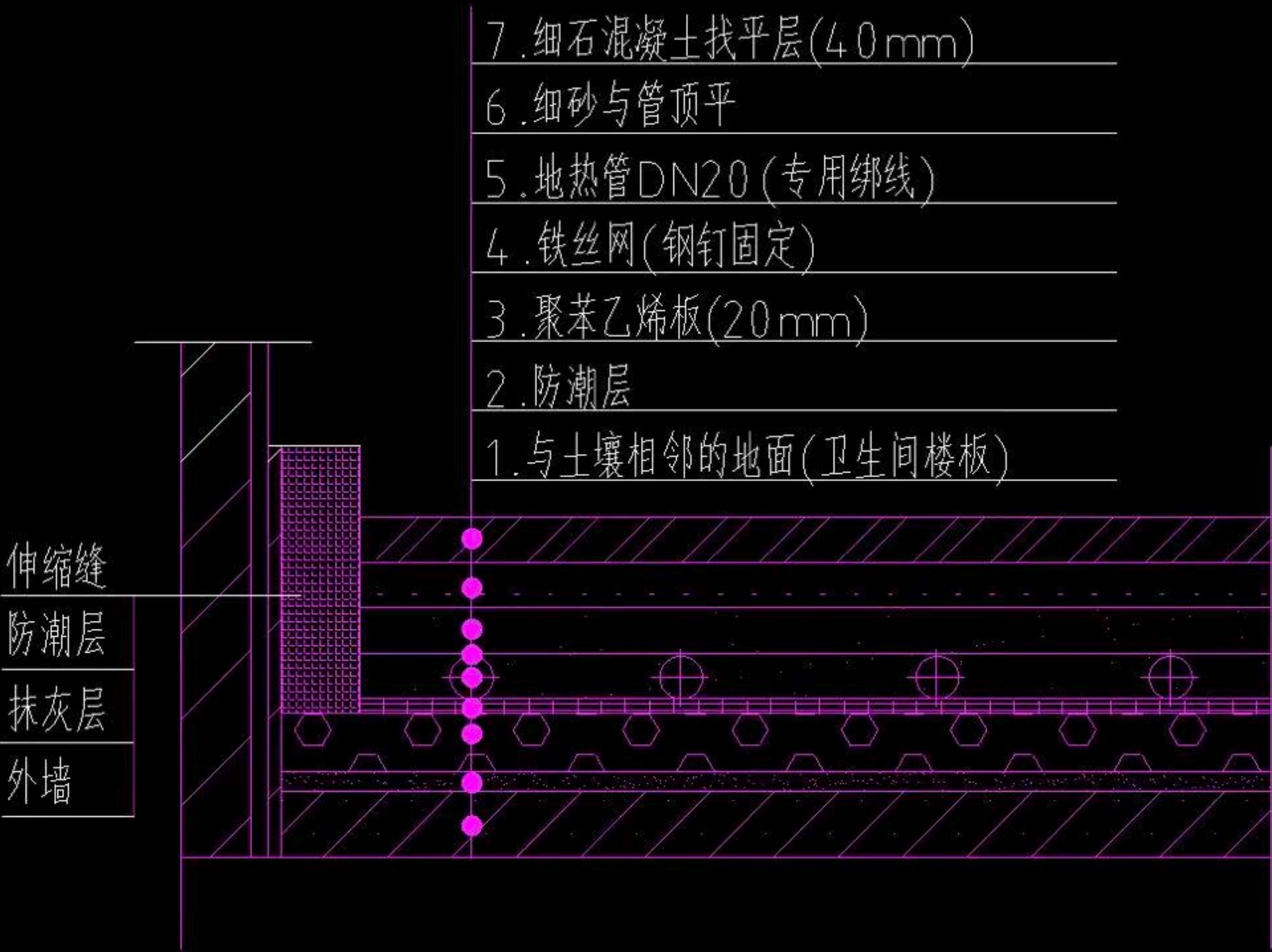
底层辐射供暖地板的构成
