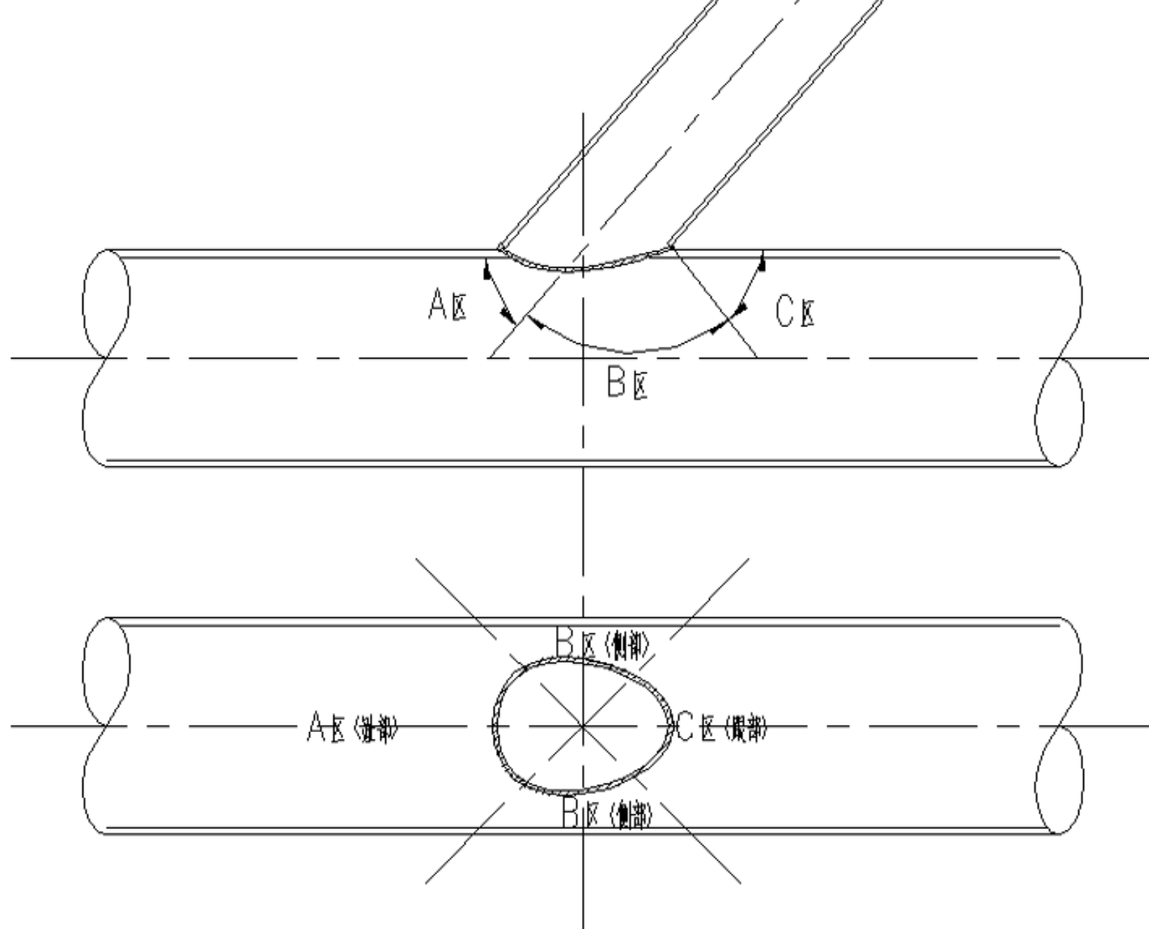
附图4 管式相贯节点焊缝分区图
