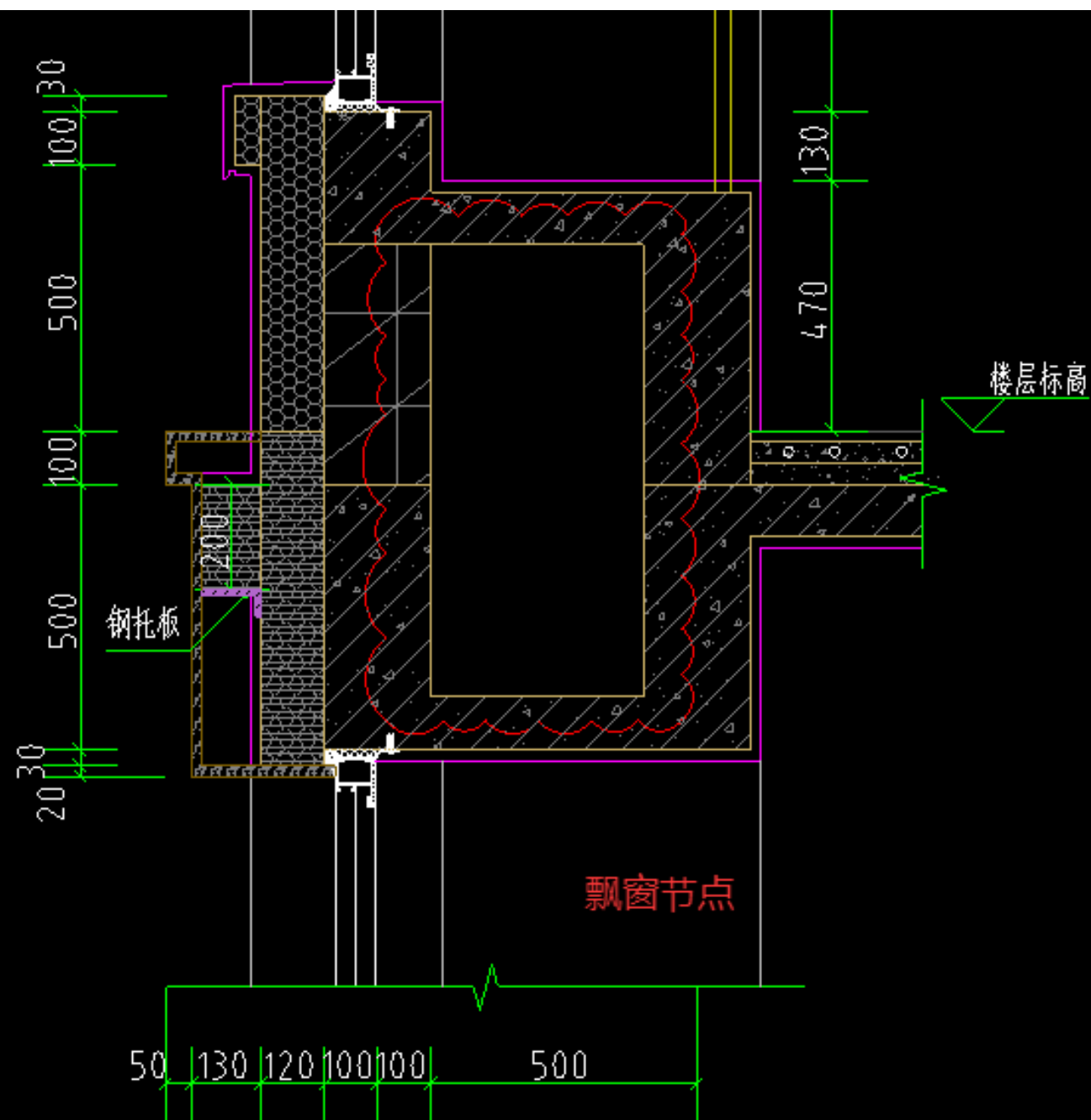
飘窗及宽窗台部位节点
